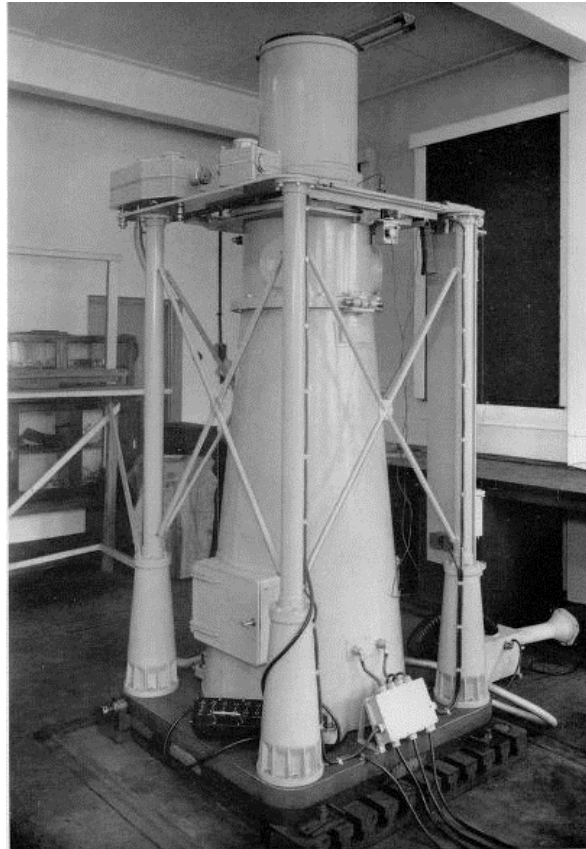
Lunette zénithale de l'Observatoire de Neuchâtel fabriquée par Grubbs, Parsons and Co. Ltd (Catalogue n°17, 1956).
