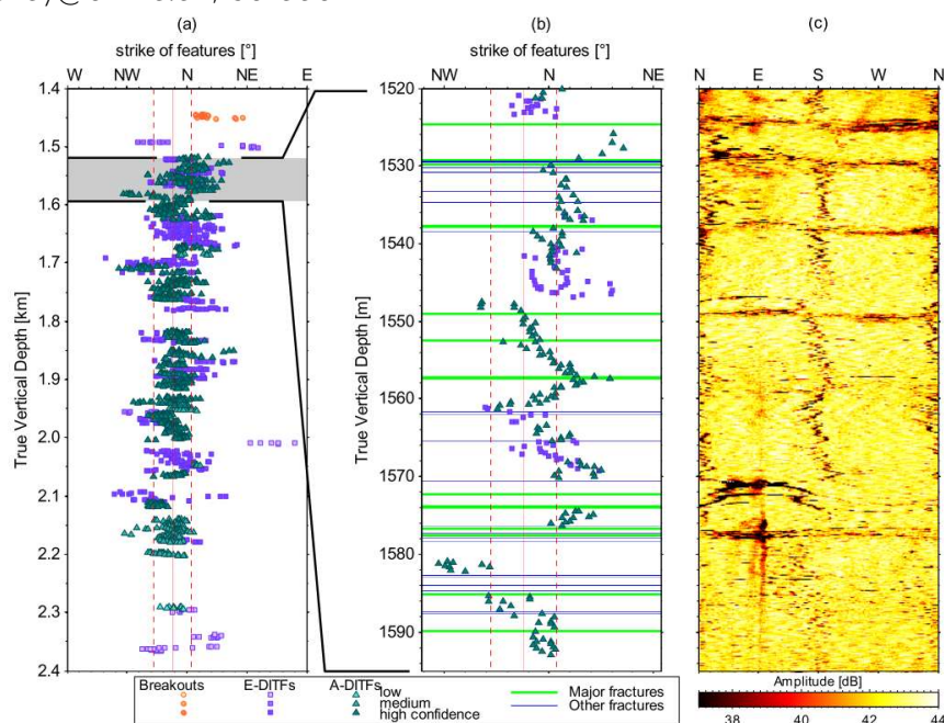
Rupture en forage soulignant la variabilité des contraintes (Valley & Evans, 2010)
