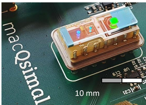
Prototype de l'horloge atomique miniature commerciale.
