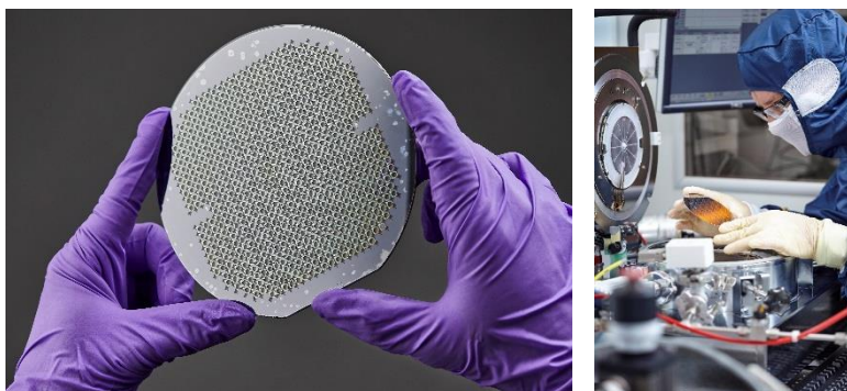
Plaquette de cellules MEMS à vapeur atomique et son développement dans les salles blanches du CSEM.
