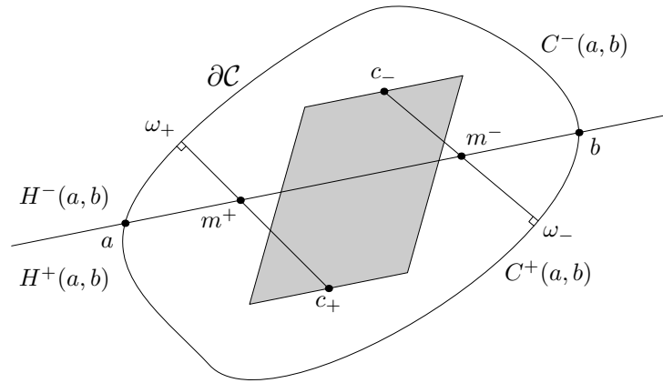
FIG. 16 — Lemme B.3 (i)
