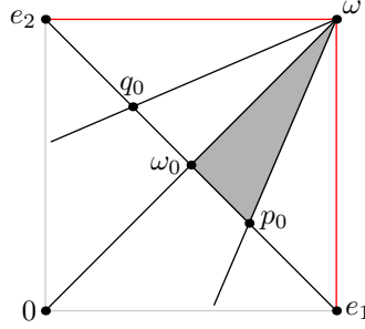
FIG. 4 – Cas d'un convexe possédant un « coin »
