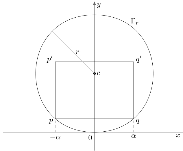
FIG. 15 – Lemme B.2
