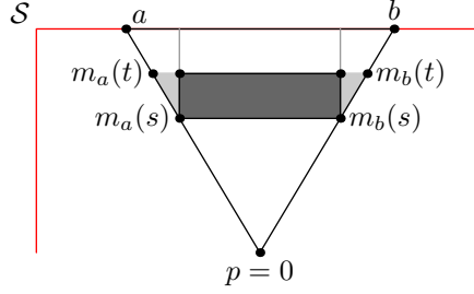
FIG. 3 – Cas d'un convexe dont le bord contient un segment
