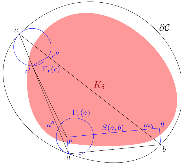
FIG. 12 – Cas où \hat{a} > \pi/2
