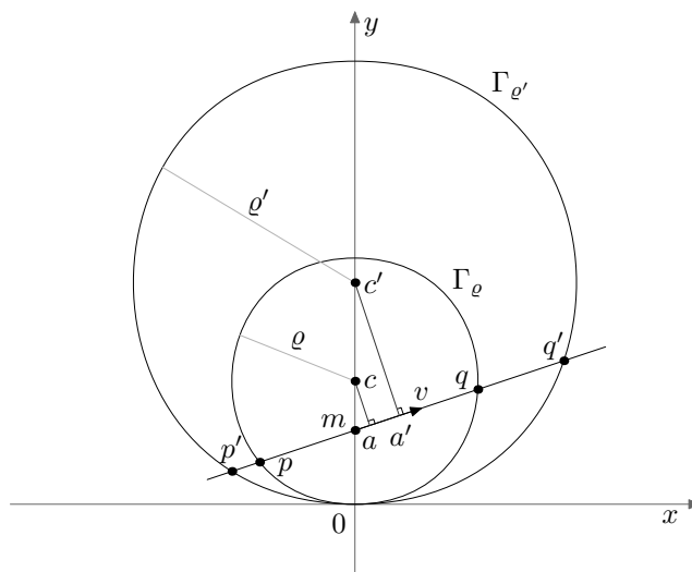
FIG. 14 – Lemme B.1
