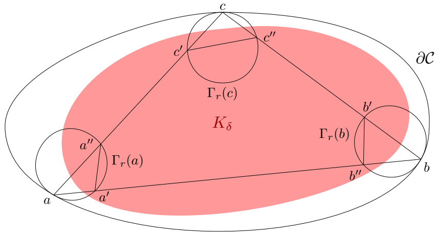
FIG. 8 – Premier cas
