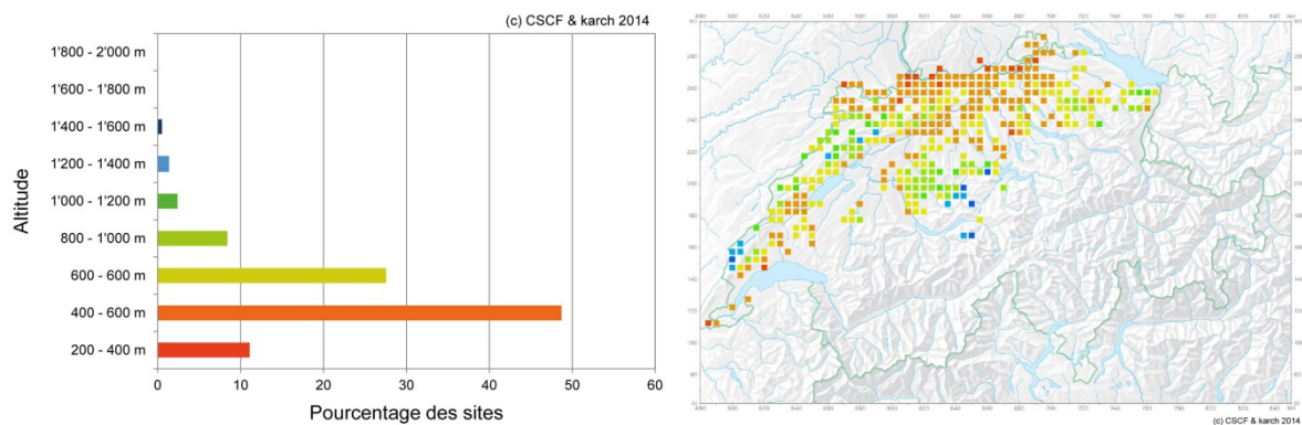
Distribution altitudinale des observations de crapaud accoucheur ( Alytes obstetricans ) en Suisse
